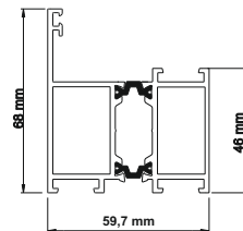
Profil proggu ENERGY 60
